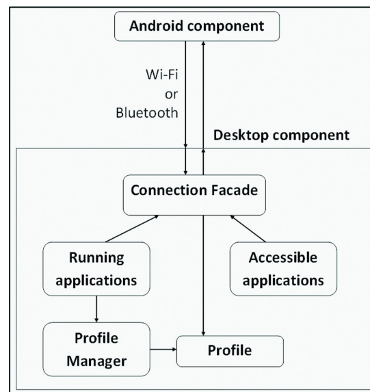
Figura 1: Arhitectura sistemului
